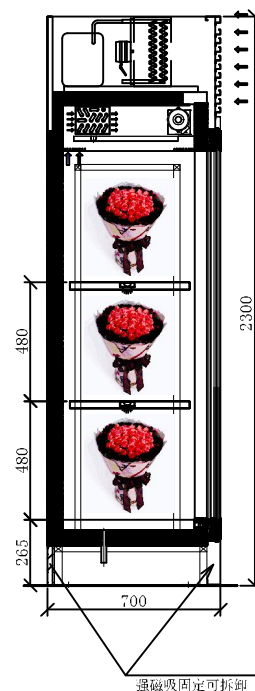
剖视图
