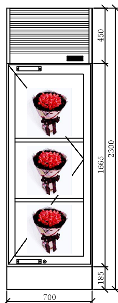
正面视图
