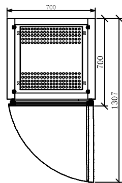
俯视图
